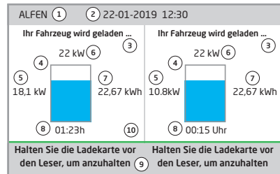
Abbildung 1b: Anzeige von Eve Double Pro-Line während des Ladevorgangs mit zwei Steckdosen
