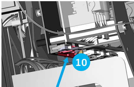
Abbildung 7: Position des SIM-Kartenhalters
