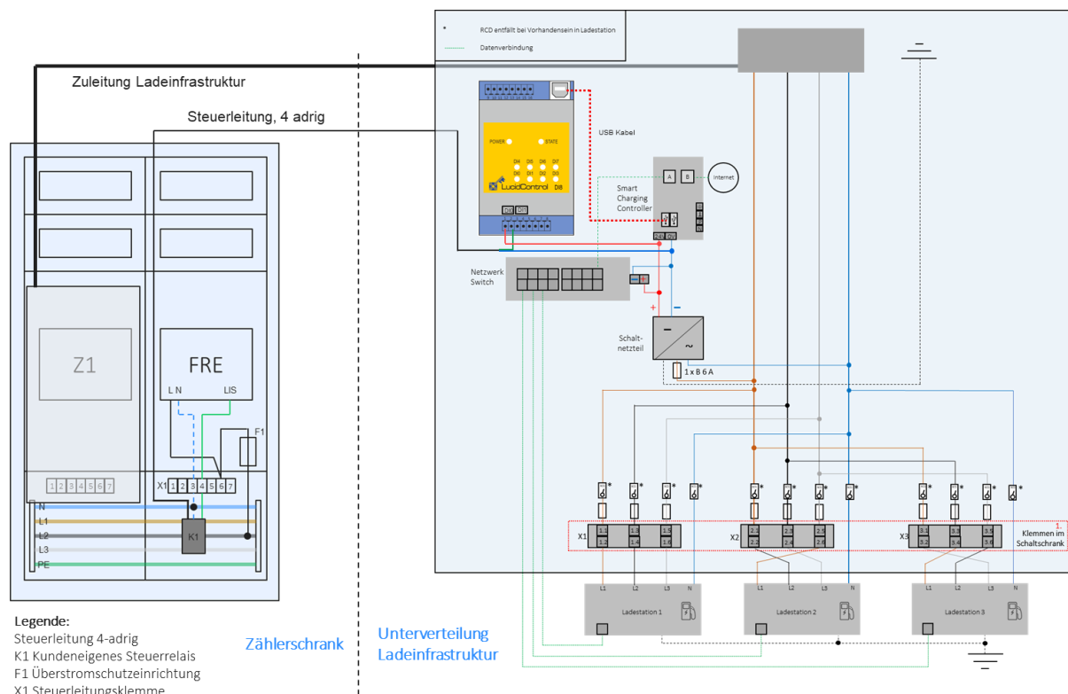
Schaltbild für eine steuerbare Verbrauchseinrichtung mit Lademanagementsystem, für den Fall einer Schaltstufe Quelle: The Mobility House GmbH
